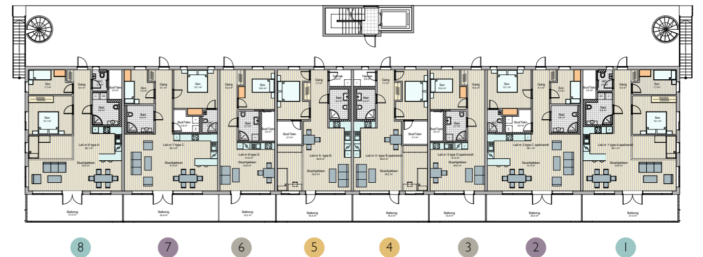
PLAN 1. ETASJE
