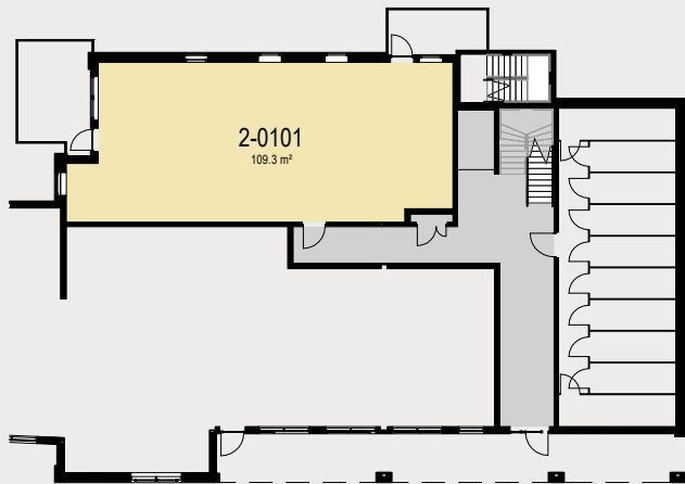
BRA 1. etg.
