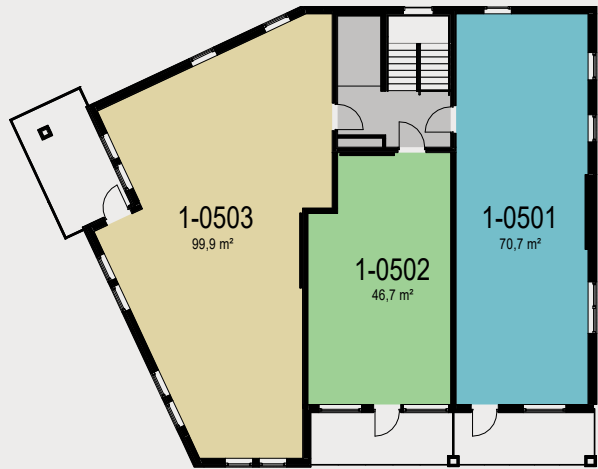
BRA 5. etg.
