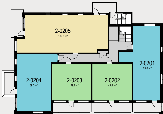
BRA 2. etg.
